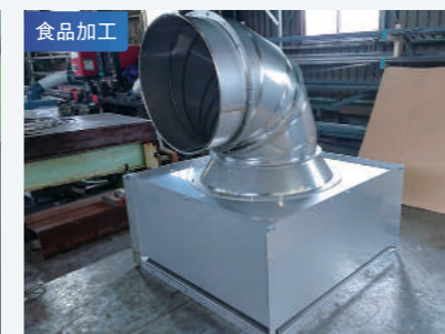
特殊ダクト
